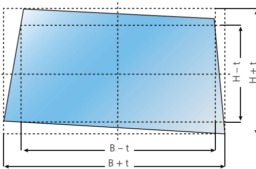
Abbildung 21: Grenzabmaße für Maße rechteckiger Scheiben
